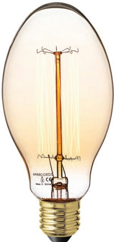
AV752 E27 25W <60 lm 2000K energy class E vetro ambrato amber glass dimmerabile dimmmable h 133mm Ø 75mm
