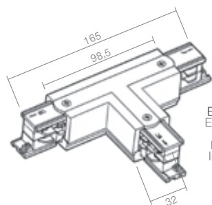
Connettore a T T Connector
